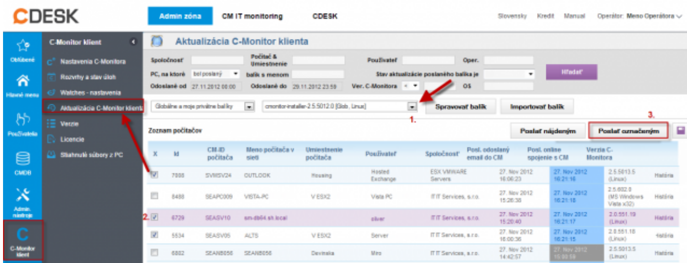
Obrázek: Rozposlanie aktualizáčného balíčka C-Monitor Linux klienta na vybrané zariadenia
